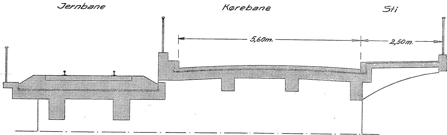
Tværsprofil visende Brobanens Inndeling ved Storstrømsbro og Oddesundbro.
