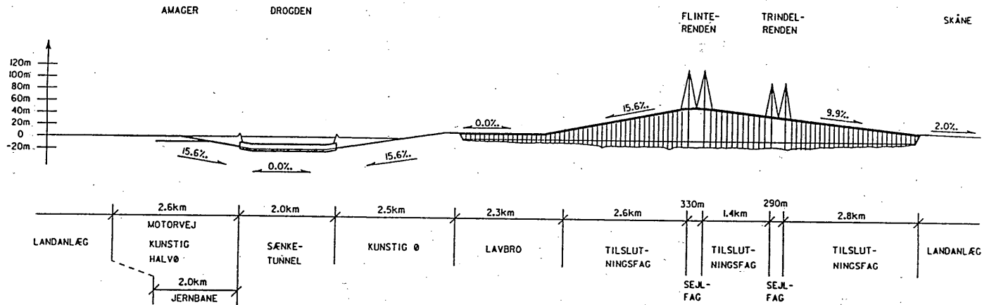
SÆNKETUNNEL
