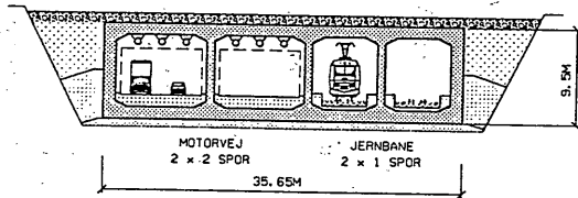
SÆNKETUNNEL
